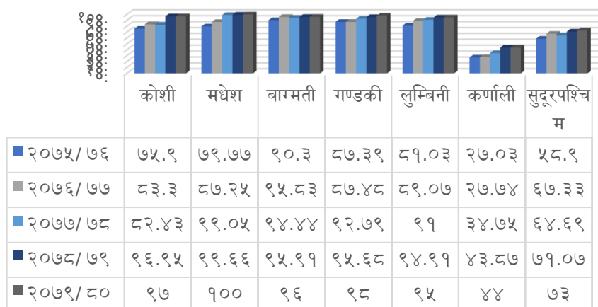
चार्ट ६.१: राष्ट्रिय प्रसारण ग्रिडबाट विद्युत पहुँच प्राप्त प्रदेशगत जनसङ्ख्या (प्रतिशतमा)
